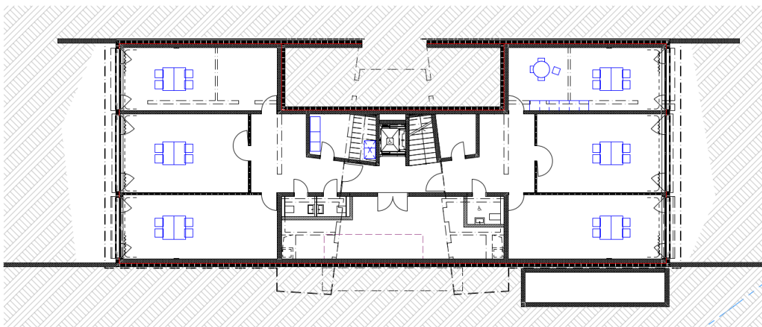
Untergeschoss (Sockelgeschoss)
