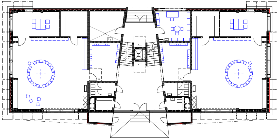
Erdgeschoss
